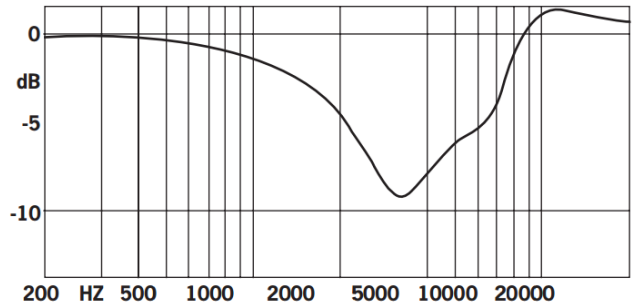
Glass Passive EQ
